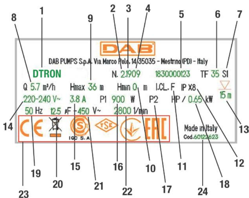
Fig.4 Targhetta
